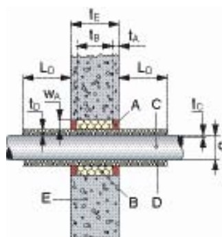
Aislamiento local no interrumpido
