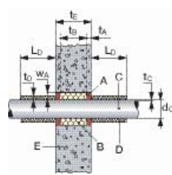
Aislamiento local interrumpido
